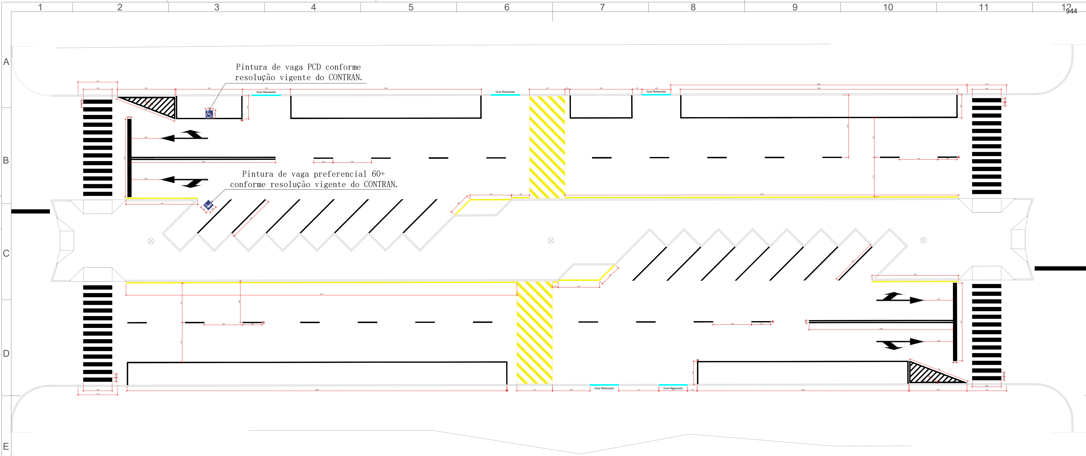
SINALIZAÇÃO HORIZONTAL – TRECHO 02 ESCALA: 1/200
