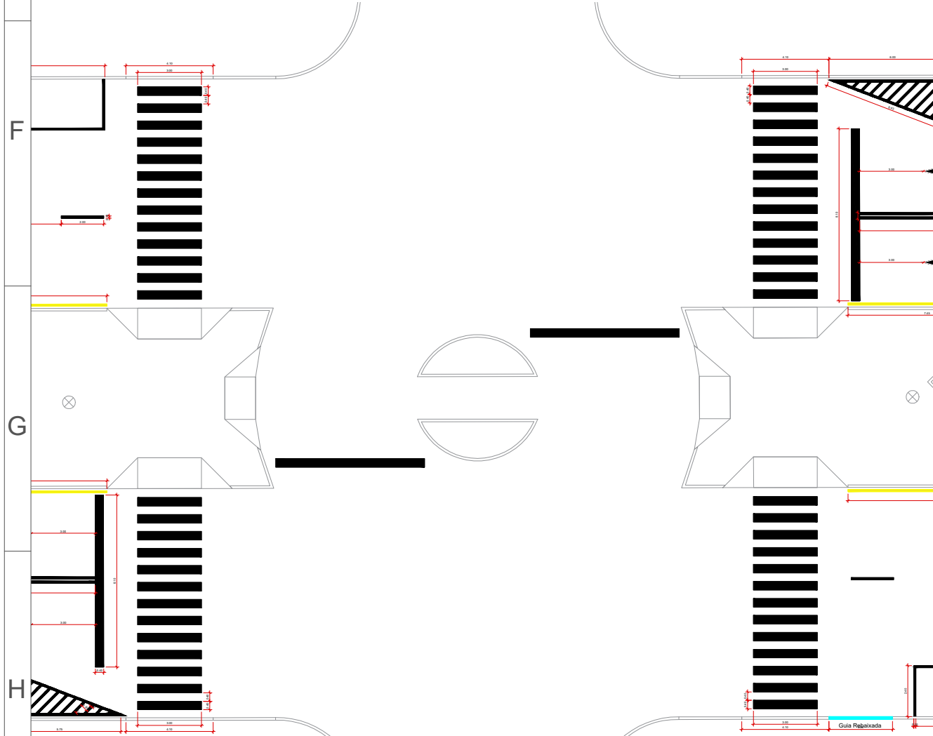
SINALIZAÇÃO HORIZONTAL – TRECHO 03 ESCALA: 1/200
