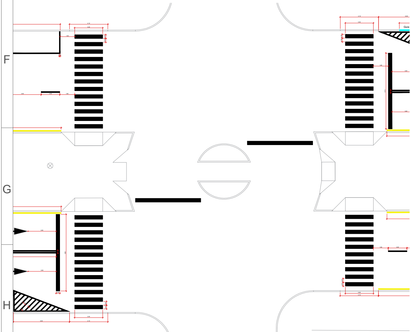
SINALIZAÇÃO HORIZONTAL – CRUZAMENTO 06 ESCALA: 1/250
