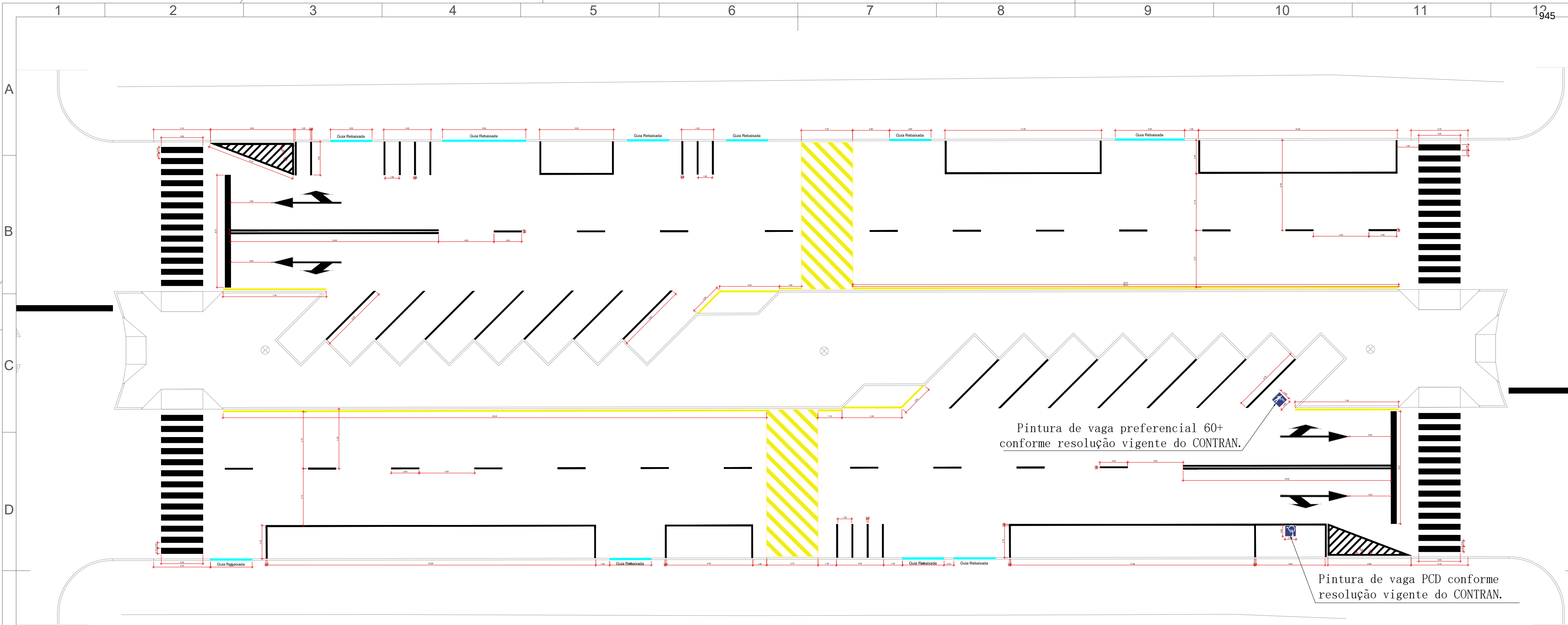
SINALIZAÇÃO HORIZONTAL – TRECHO 03 ESCALA: 1/200
