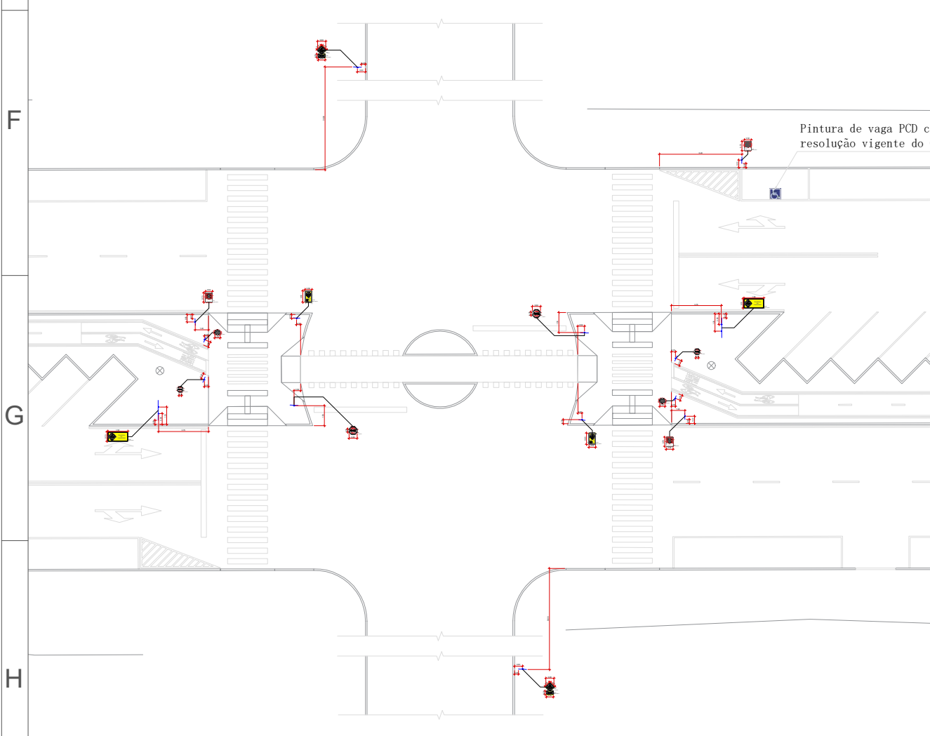
SINALIZAÇÃO VERTICAL – CRUZAMENTO 01 ESCALA: 1/400
