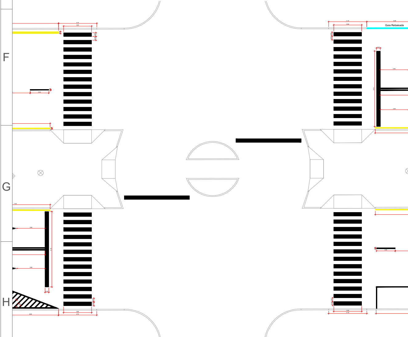
SINALIZAÇÃO HORIZONTAL – CRUZAMENTO 04 ESCALA: 1/250
