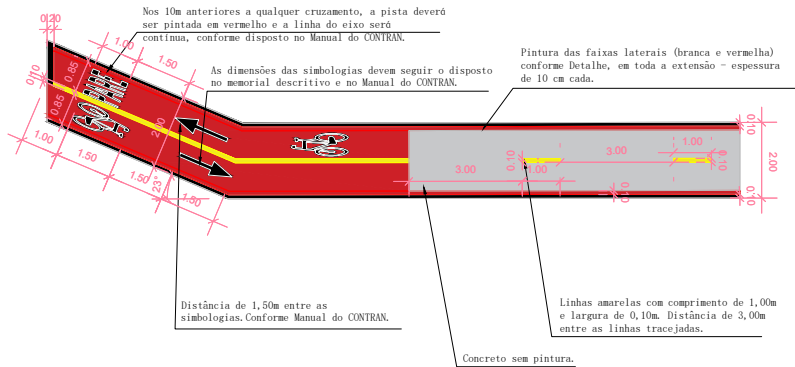
DETALHE CICLOVIA ESCALA: 1/200
