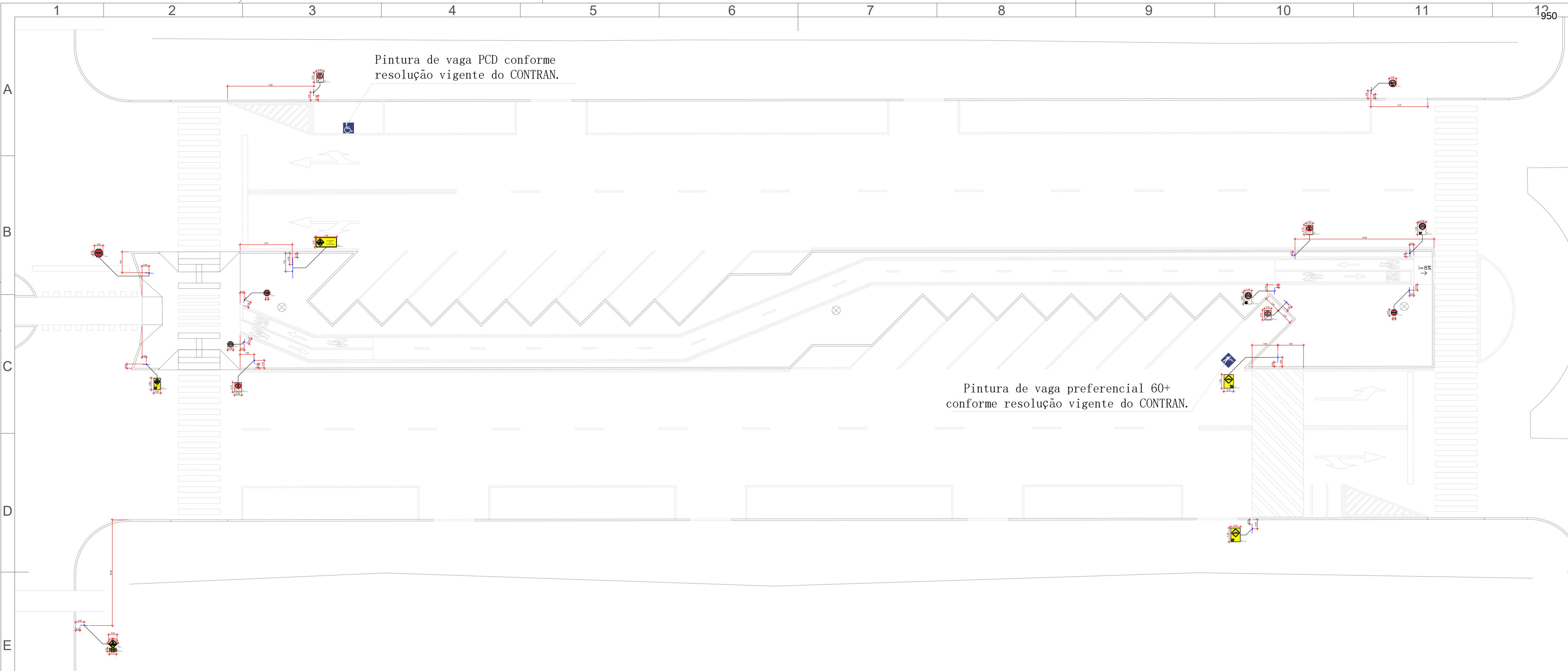
SINALIZAÇÃO VERTICAL – TRECHO 01 ESCALA: 1/200
