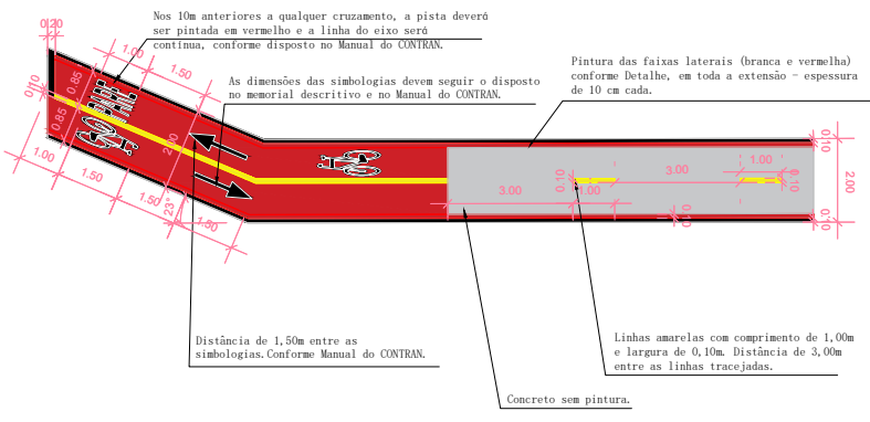
DETALHE CICLOVIA ESCALA: 1/200
