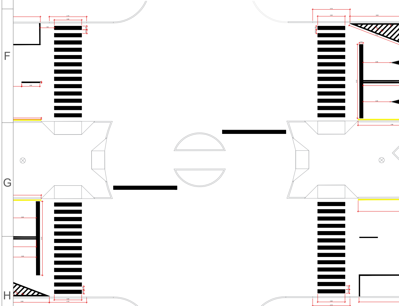
SINALIZAÇÃO HORIZONTAL – CRUZAMENTO 02 ESCALA: 1/250
