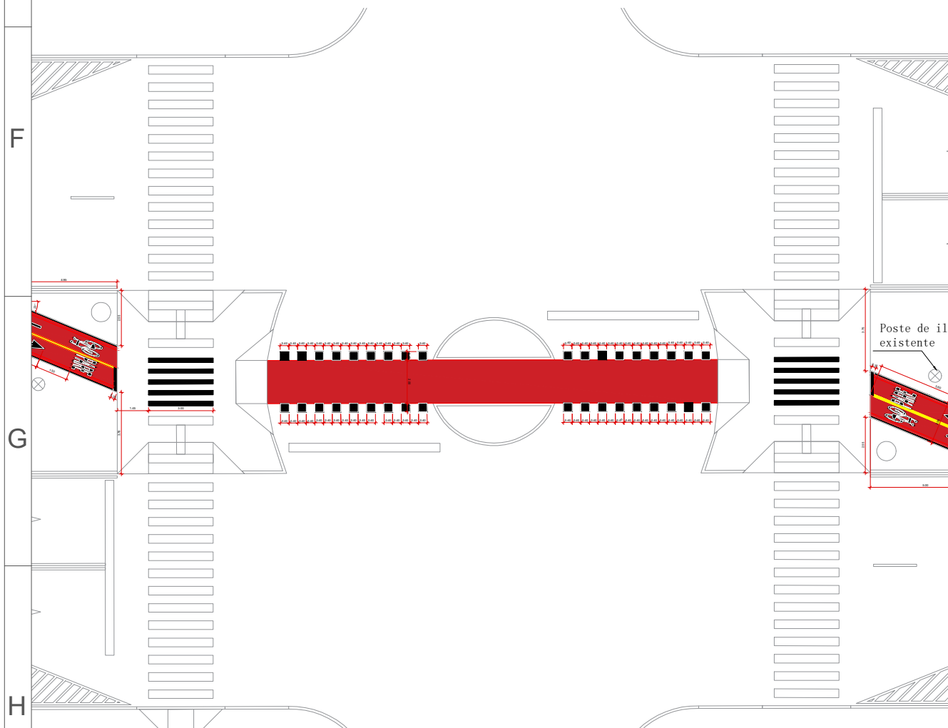
CICLOVIA – TRECHO 01 ESCALA: 1/200
