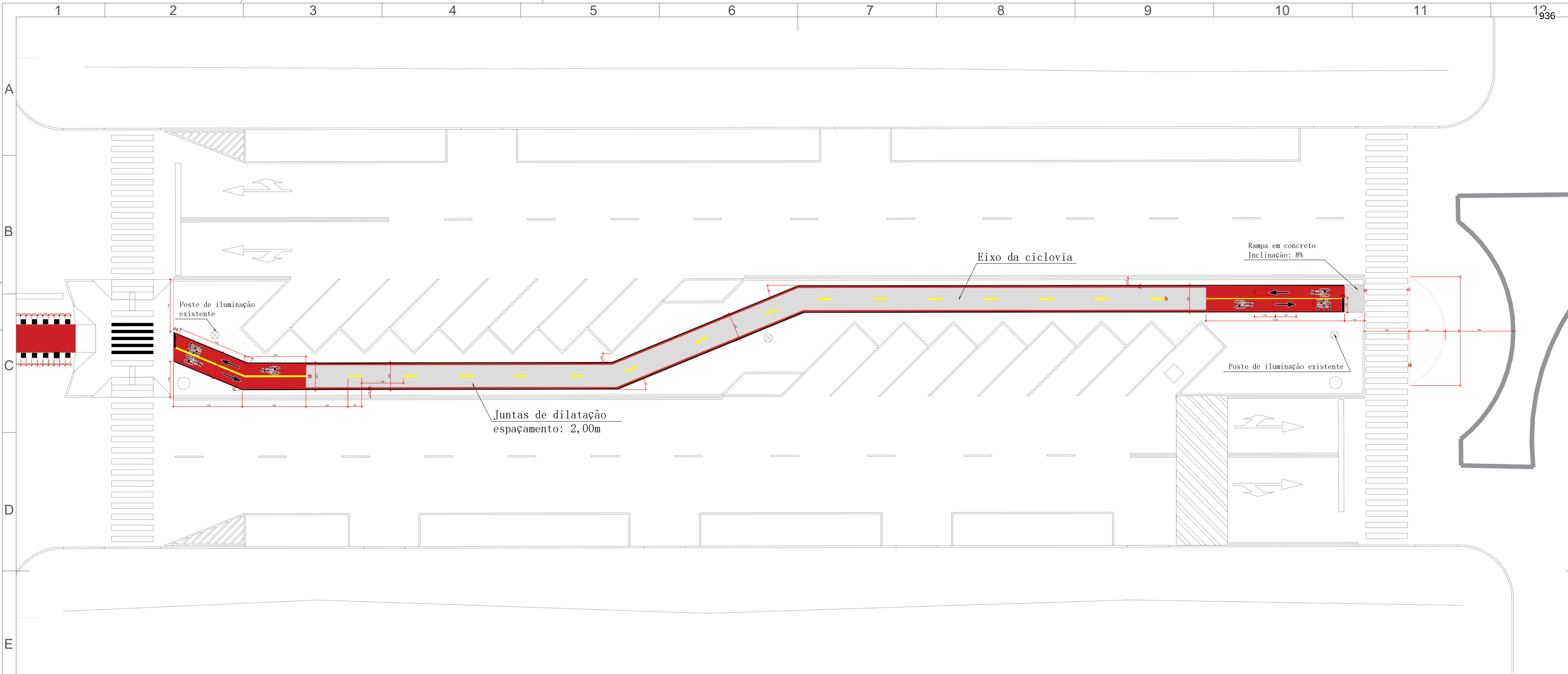
CICLOVIA – TRECHO 01 ESCALA: 1/200
