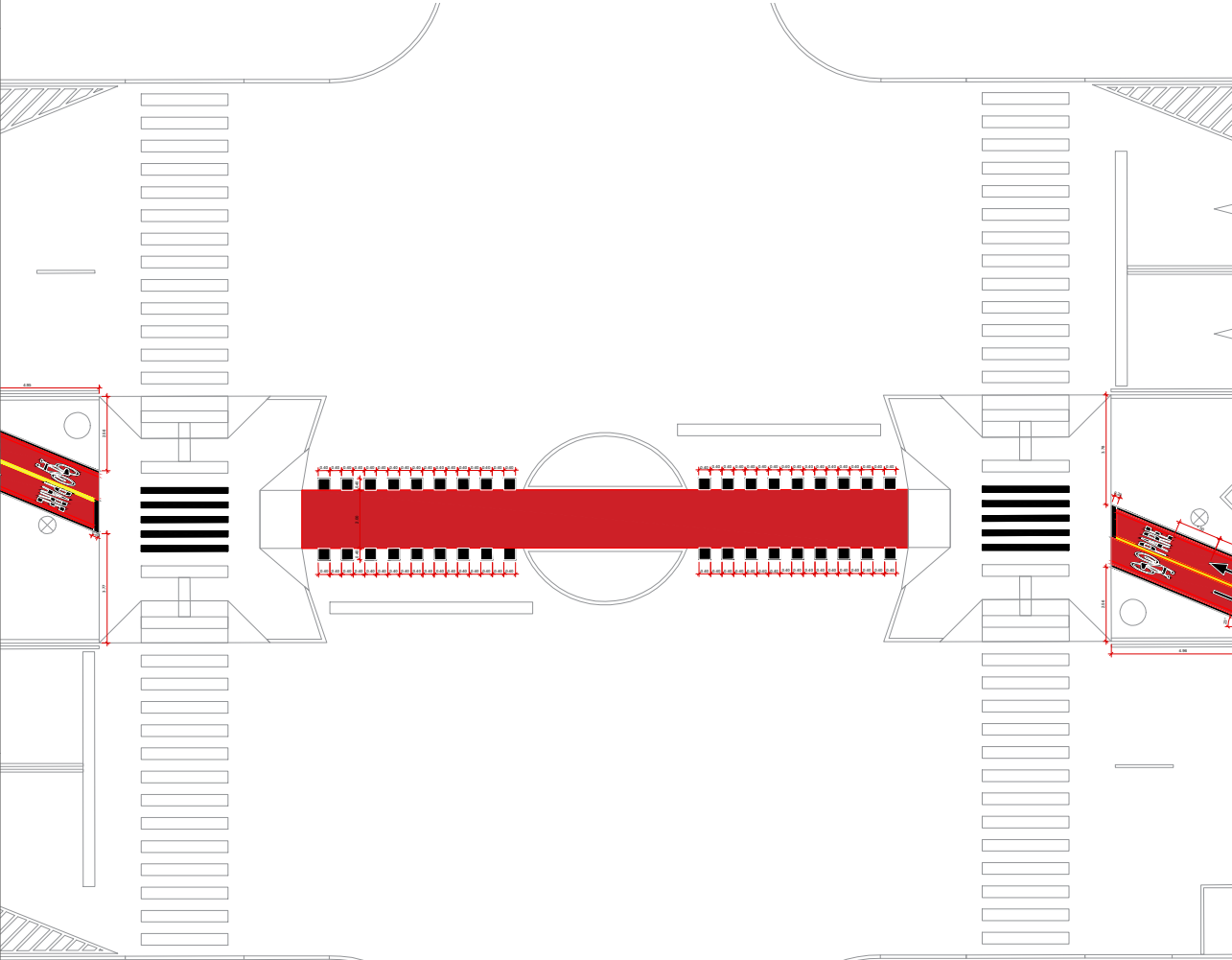
CICLOVIA – TRECHO 03 ESCALA: 1/200
